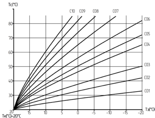
Рисунок 25 Компенсаційні криві
